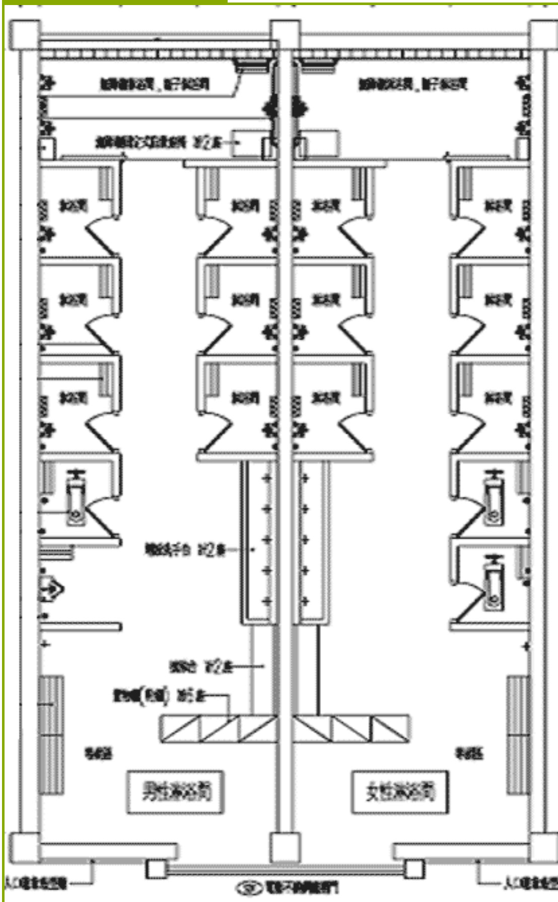
更衣淋浴間平面圖A
