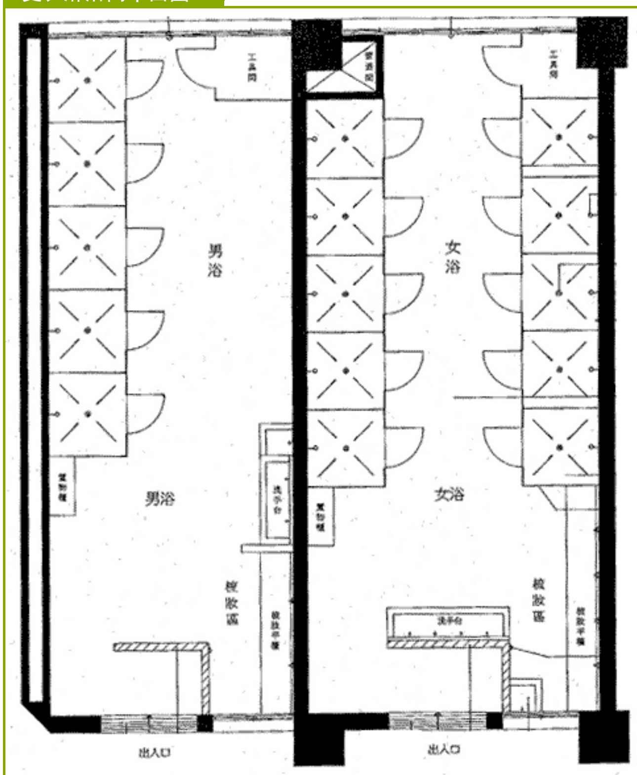
更衣淋浴間平面圖A
