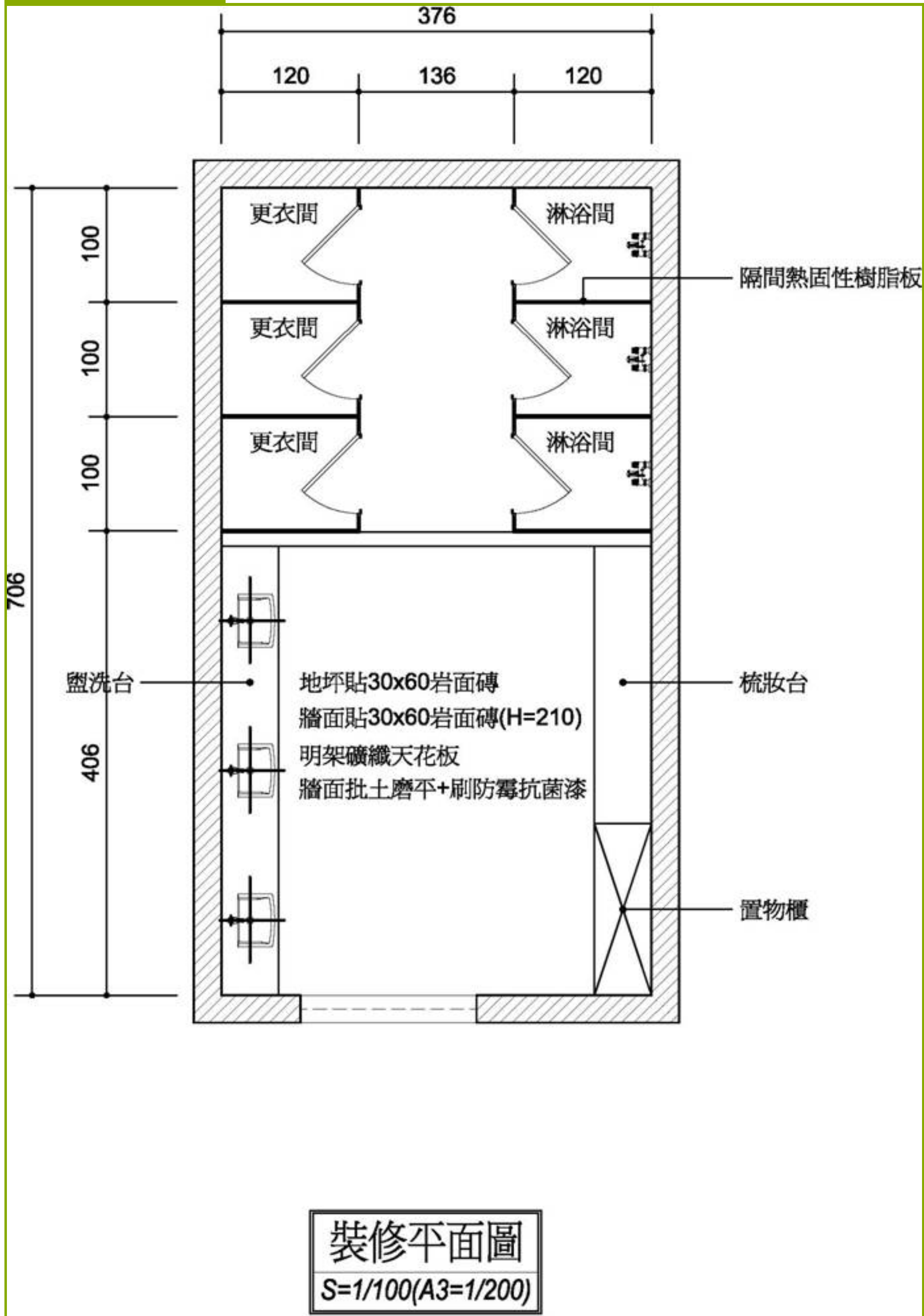
更衣淋浴間平面圖A
