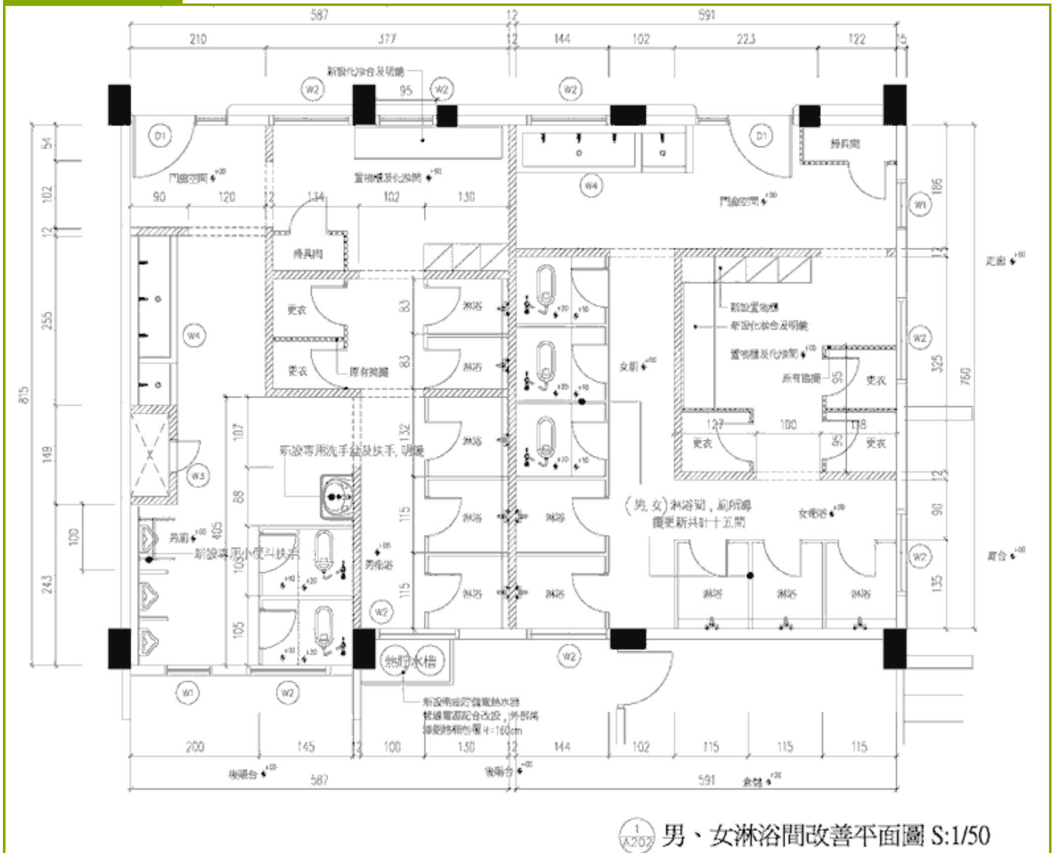
淋浴間平面圖A
