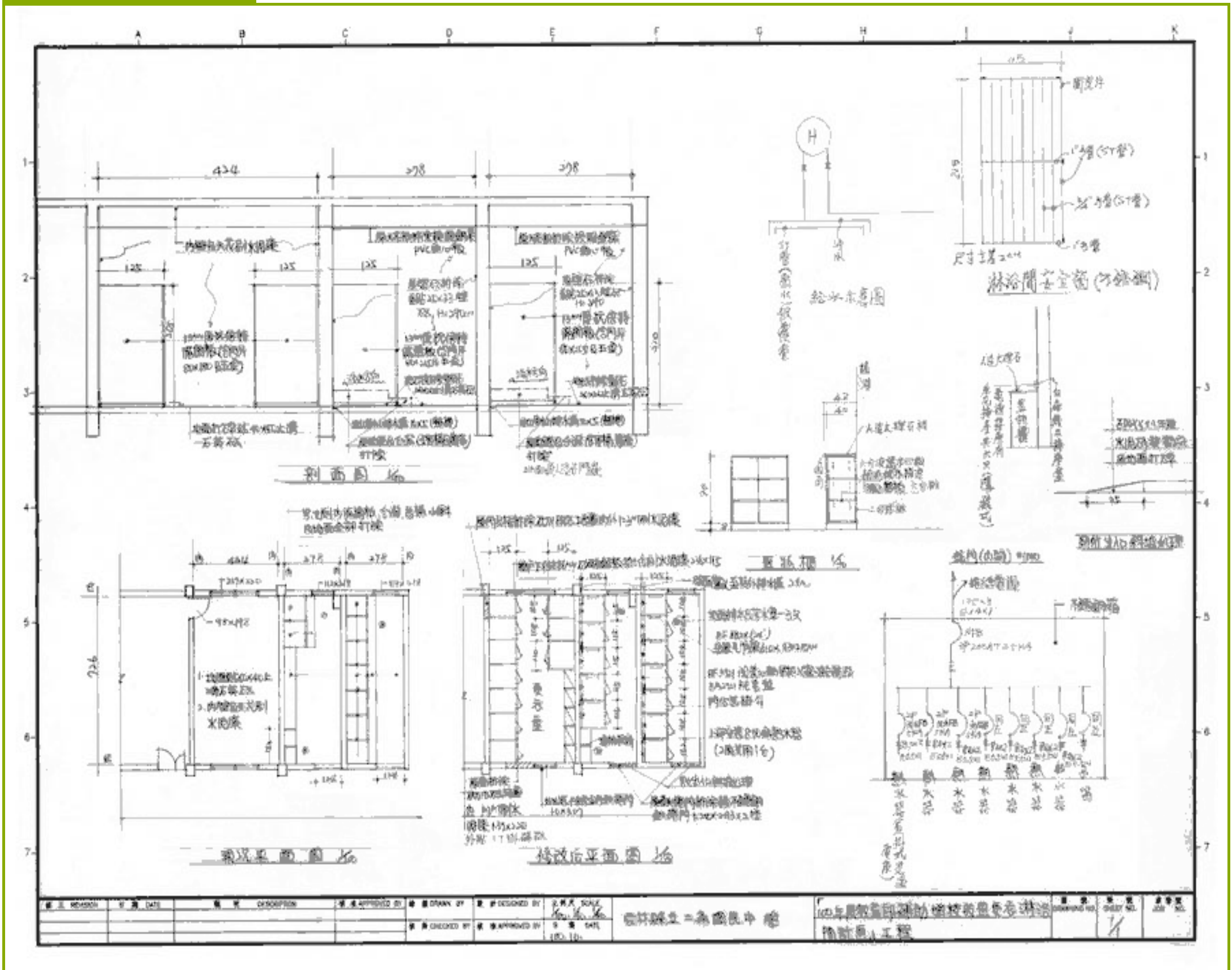
更衣淋浴間平面圖A
