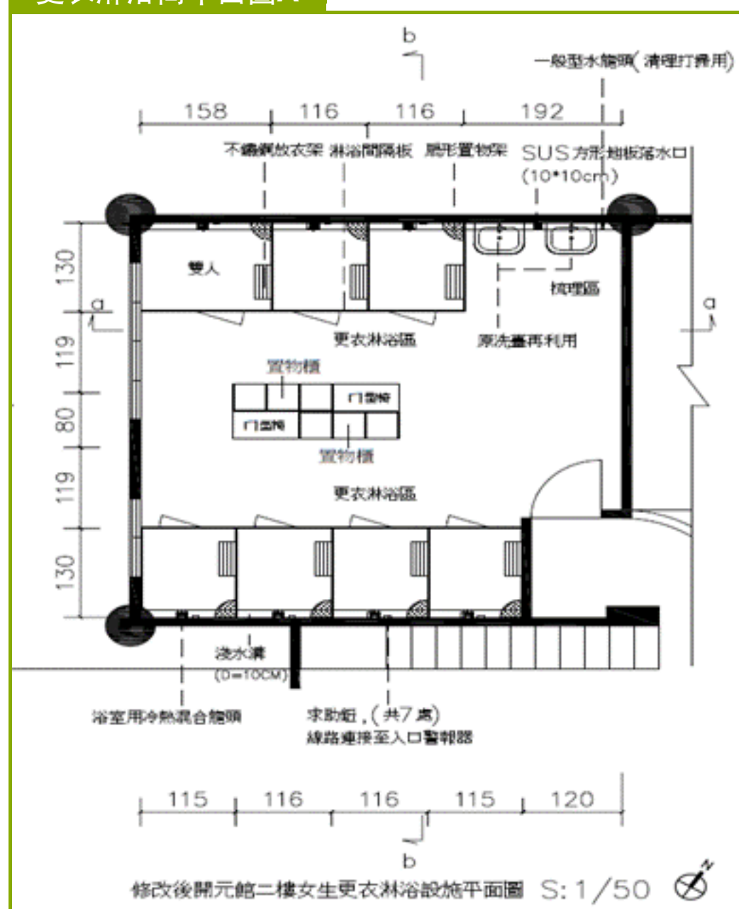
更衣淋浴間平面圖A
