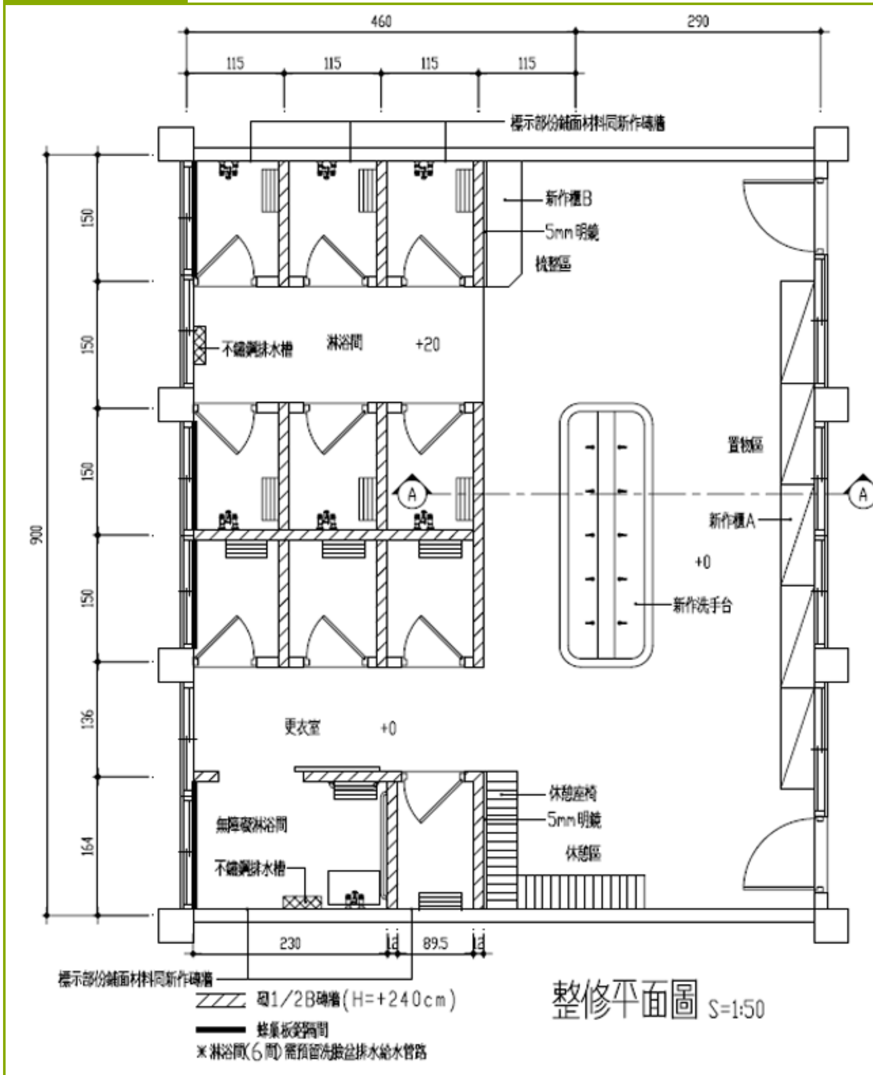
淋浴間平面圖A
