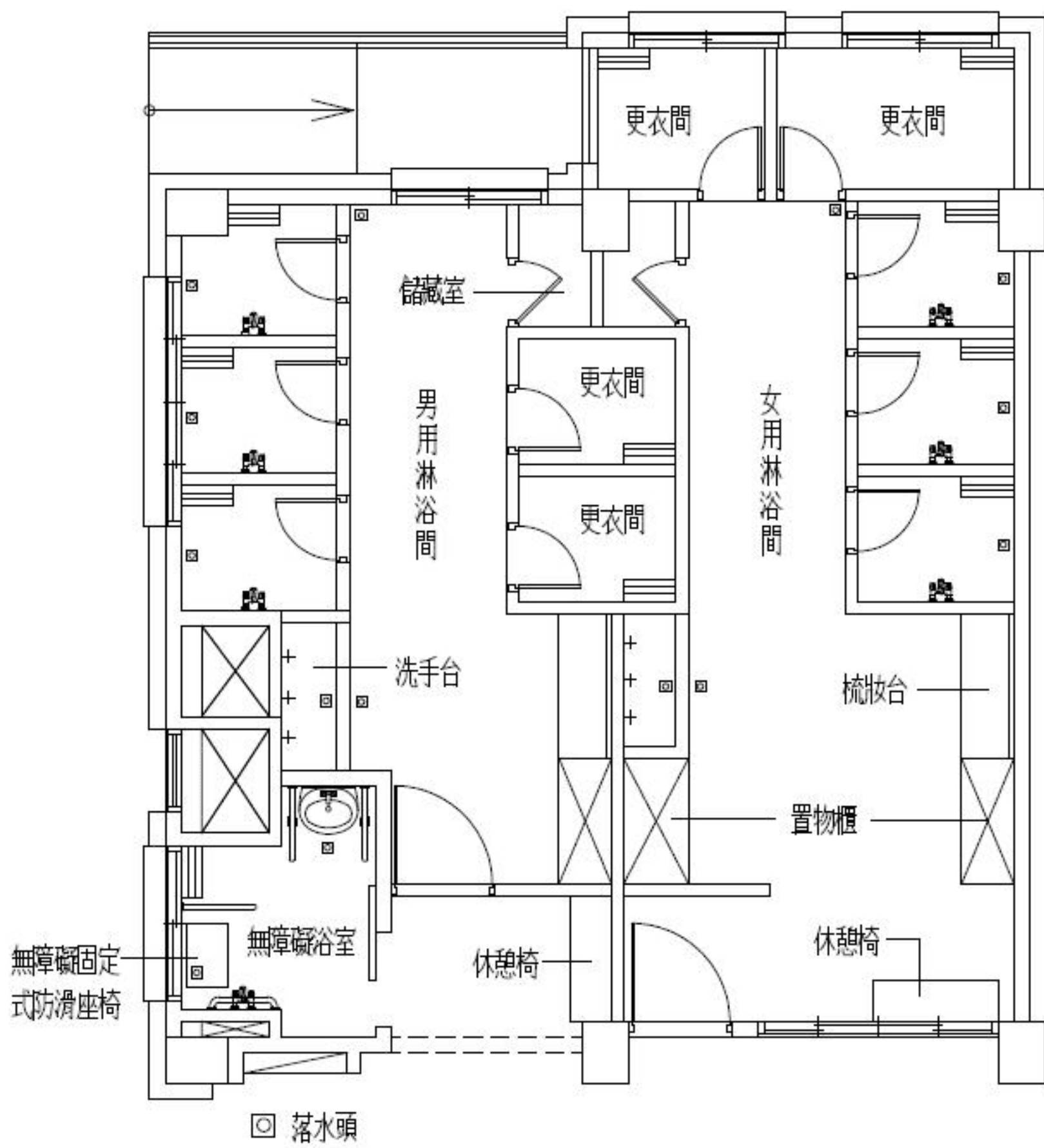
淋浴間平面配置圖 S=1:50
