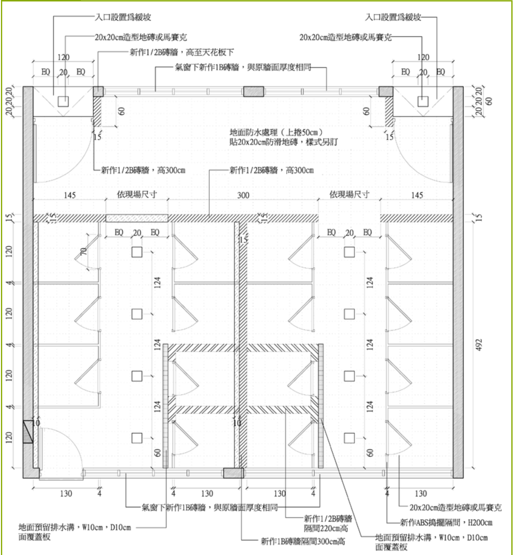
淋浴間平面圖
