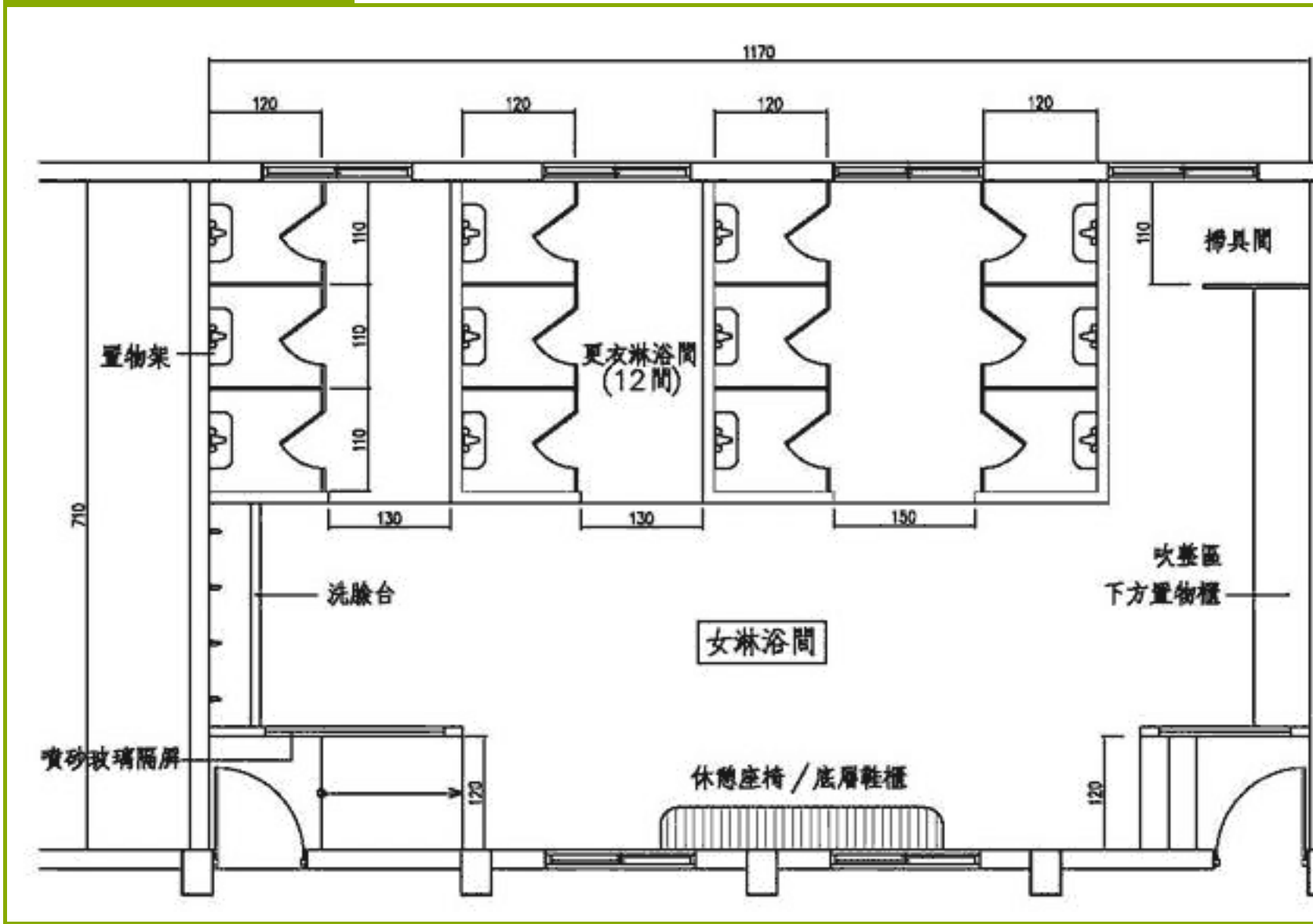
更衣淋浴間平面圖A
