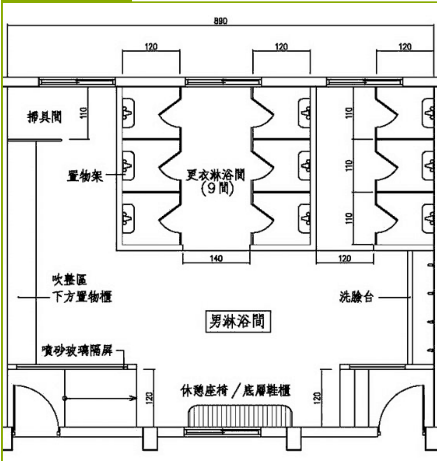
更衣淋浴間平面圖B
