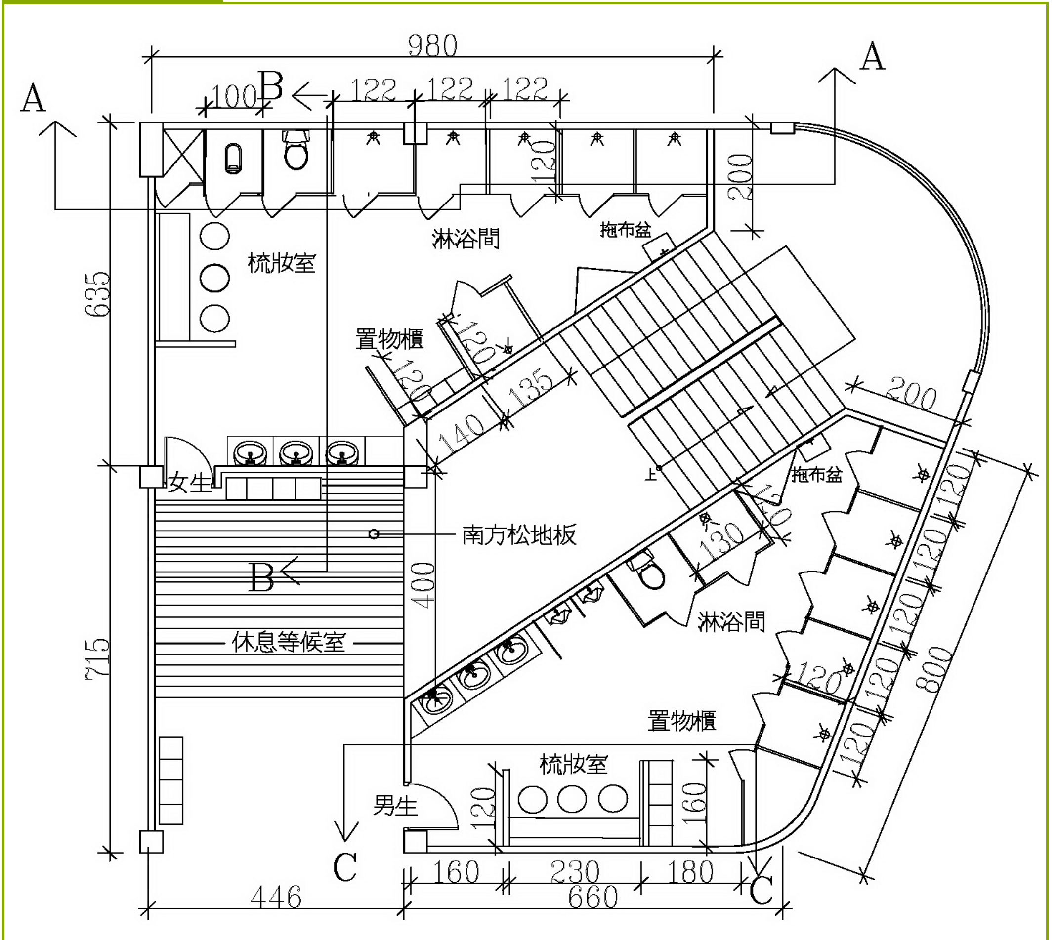
更衣淋浴間平面圖A
