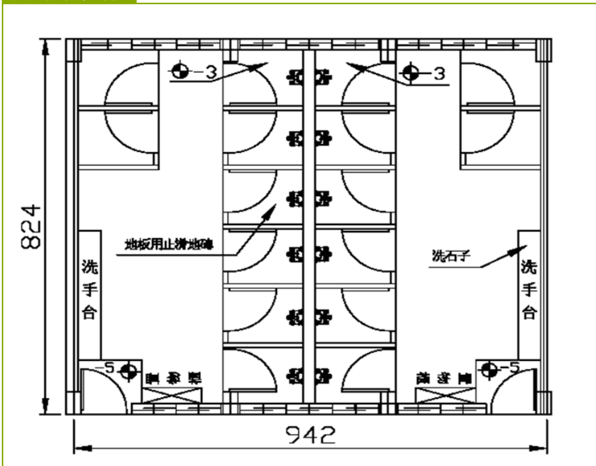
更衣淋浴間平面圖A
