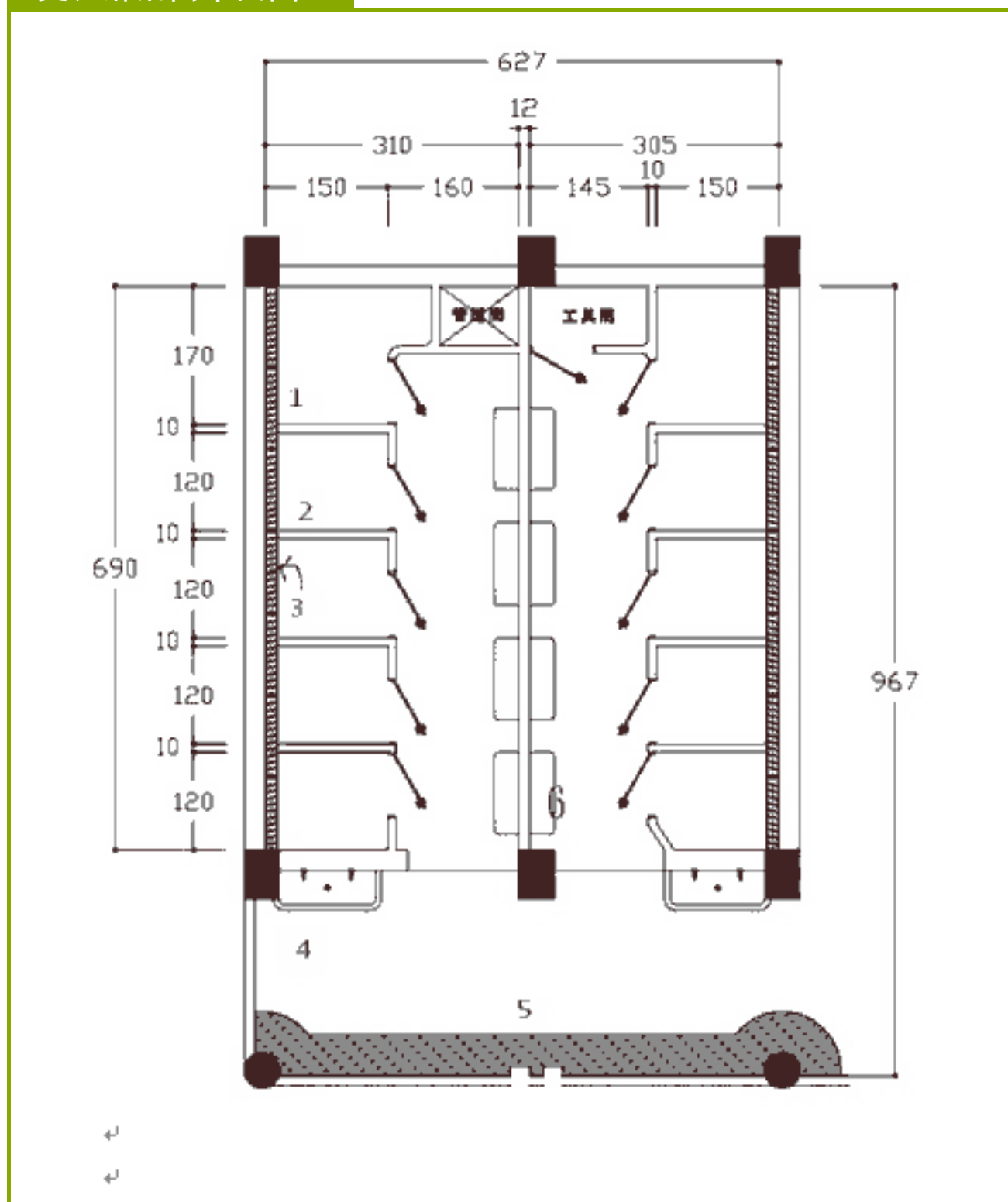
更衣淋浴間平面圖A
