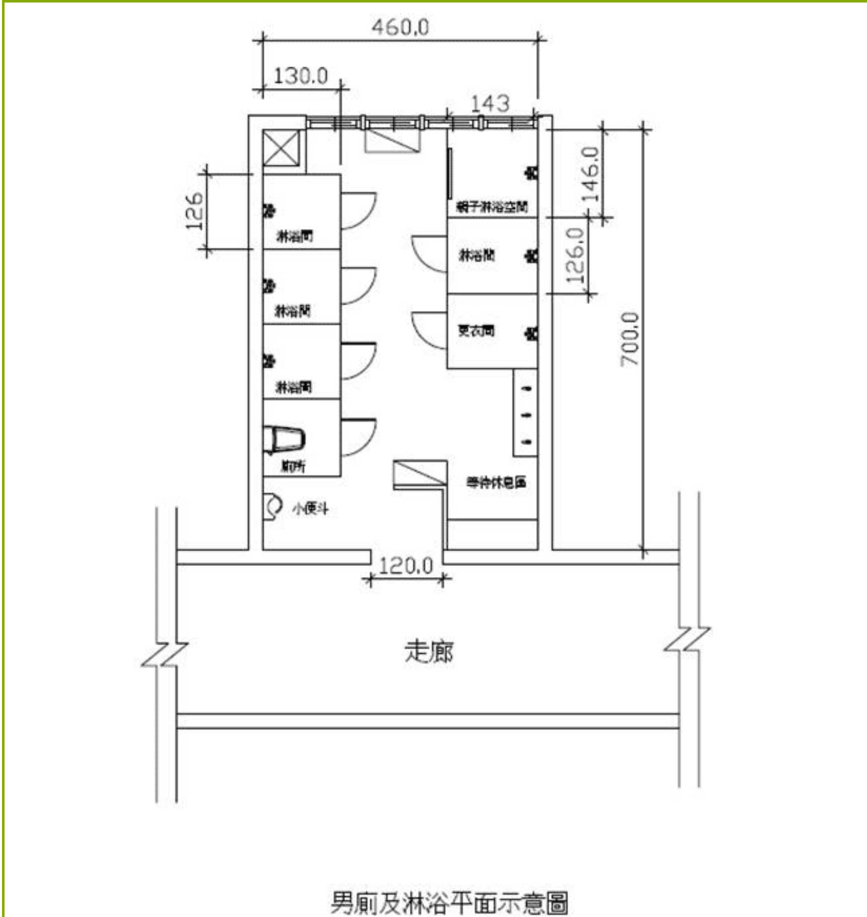
更衣淋浴間平面圖A
