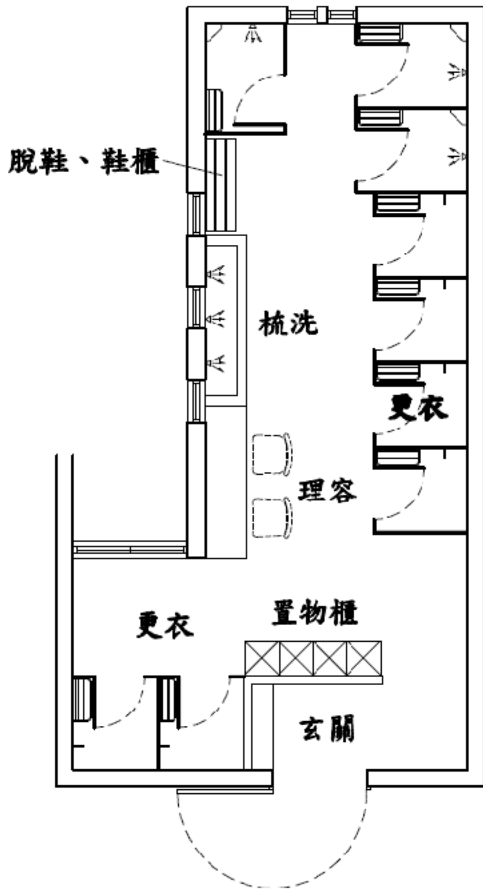
二樓女用浴室平面
