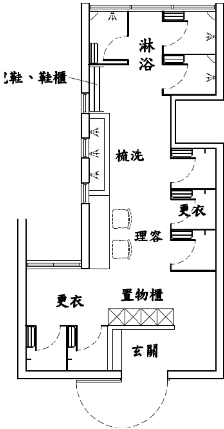
一樓男用浴室平面
