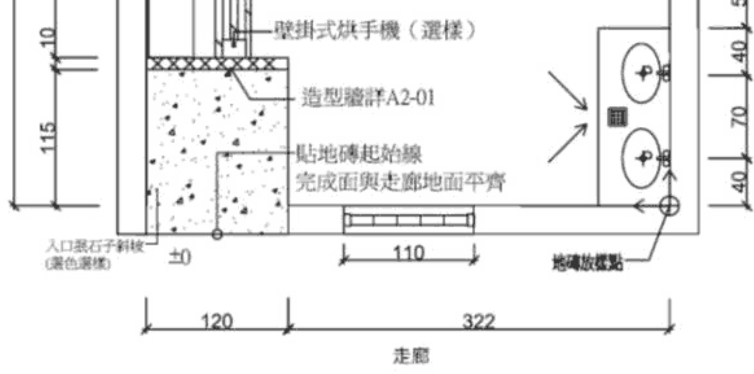
① 二樓男淋浴間整修平面圖
