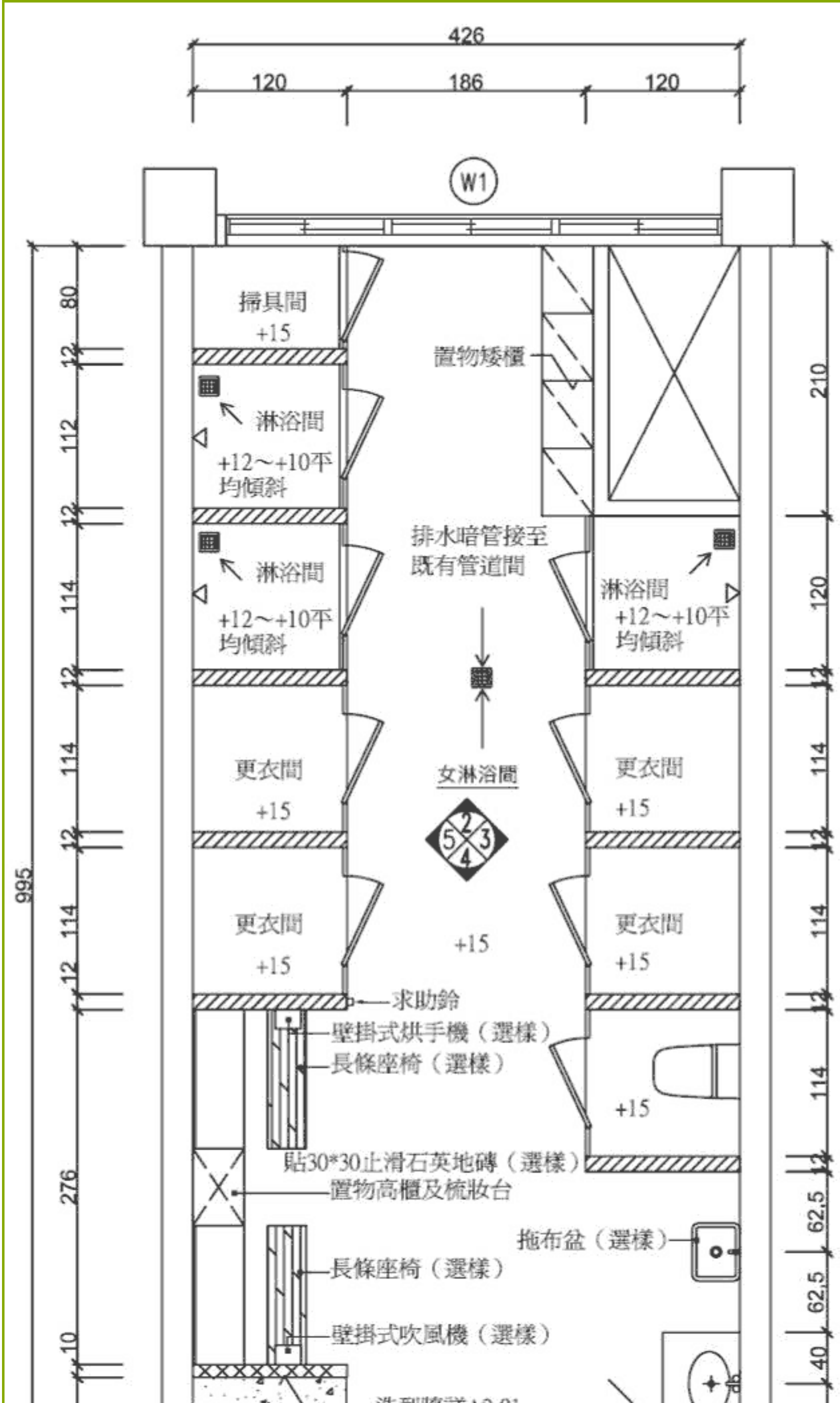
更衣淋浴間平面圖A
