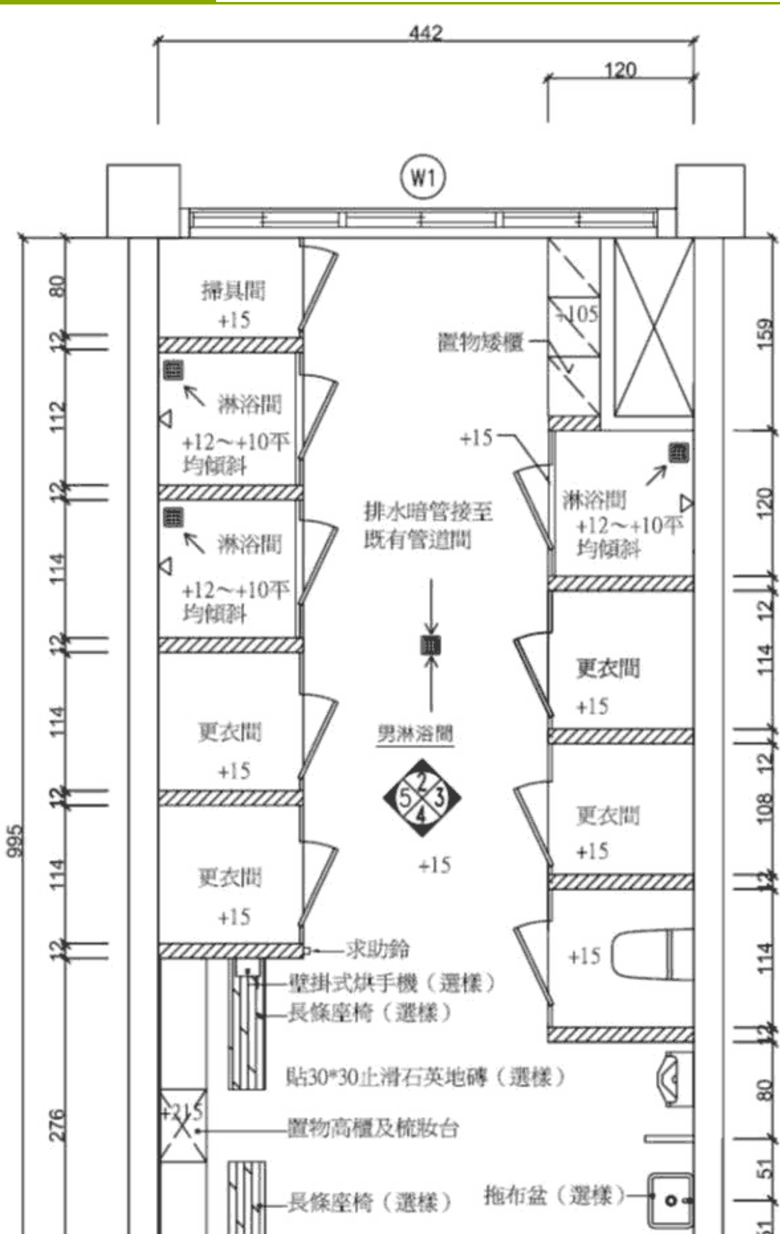
更衣淋浴間平面圖B
