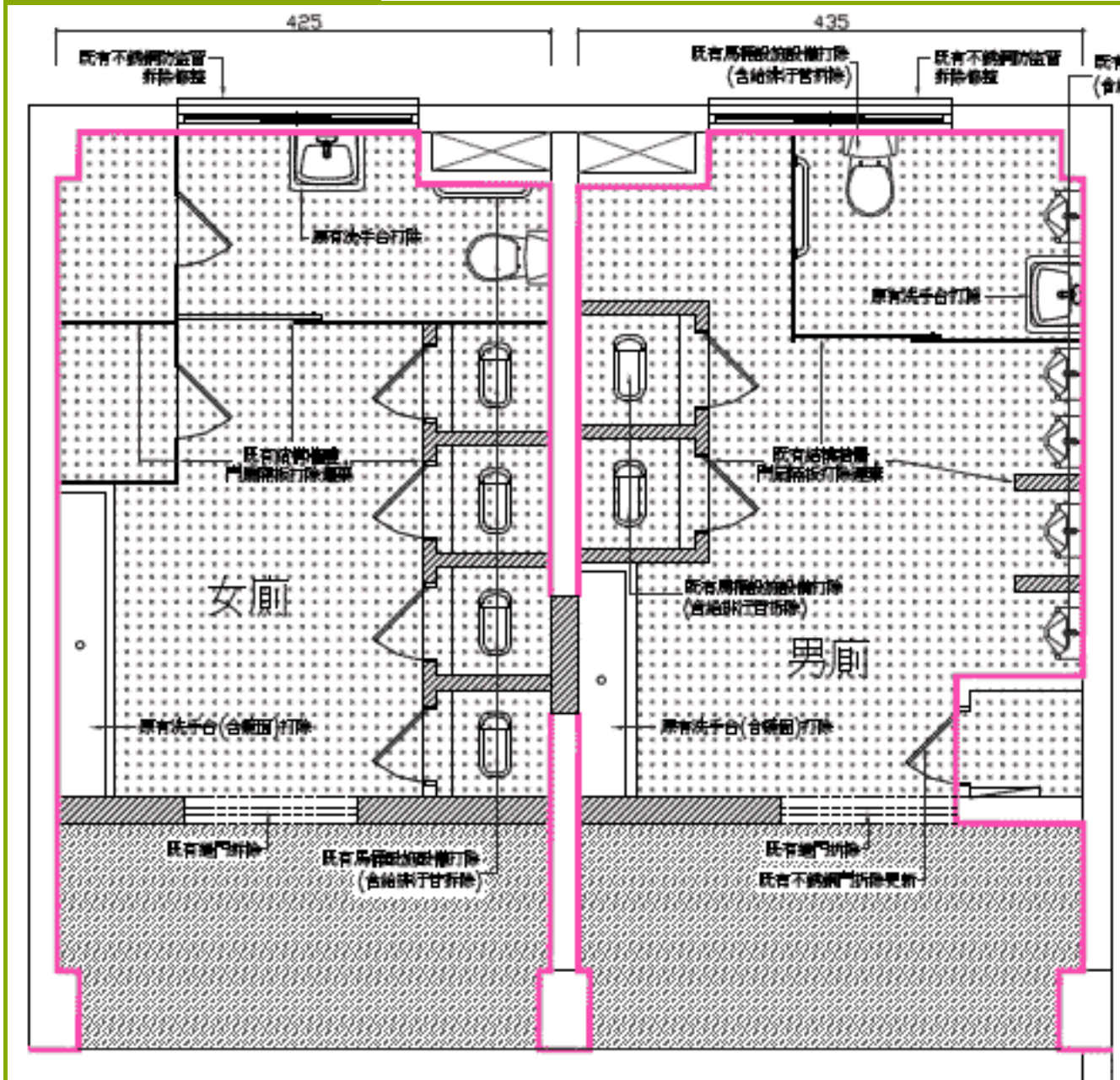
更衣淋浴間平面圖A
