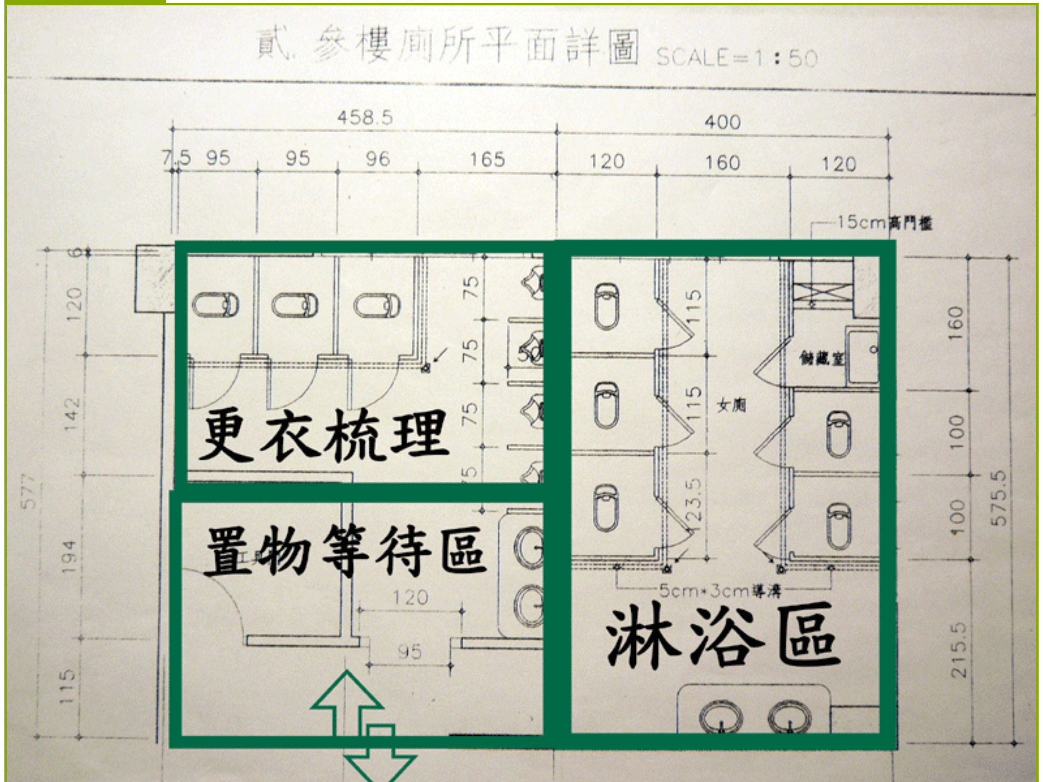
淋浴間平面圖
