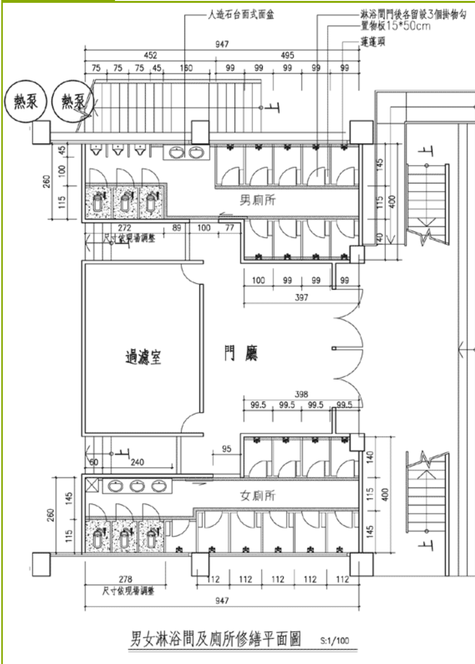
淋浴間平面圖A
