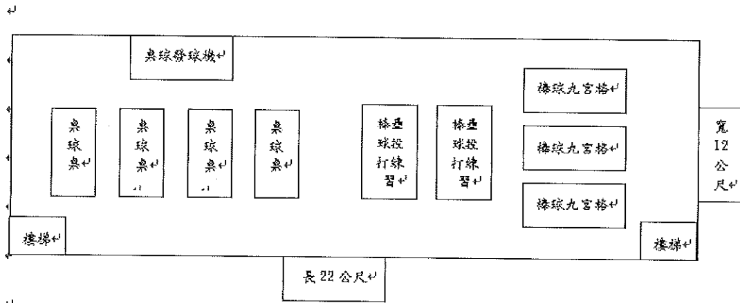
圖一 地下室運動樂活站空間尺寸與設施擺放示意圖
